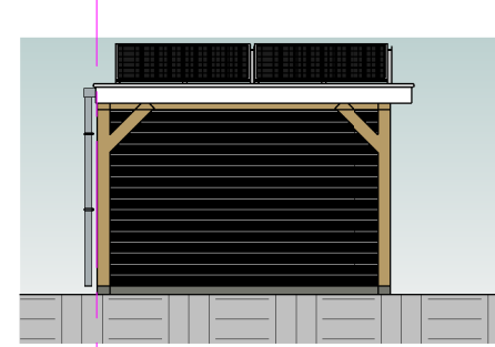
Linkergevel
